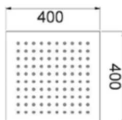
ART. SD4002A/400 FLAT Soffione doccia QUADRO 6mm INOX
