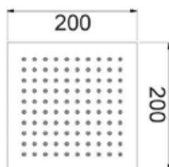
ART. SD4002A/200 FLAT Soffione doccia QUADRO 6mm INOX
