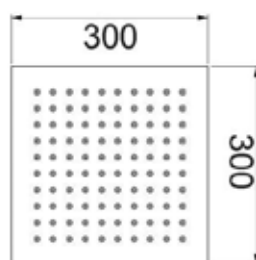
ART. SD4002A/300 FLAT Soffione doccia QUADRO 6mm INOX
